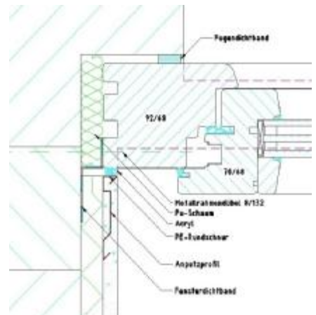
Horizontalschnitt der Anschlusssituation
