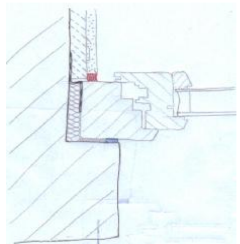
Diskussionsskizze zum Fensteranschluss
